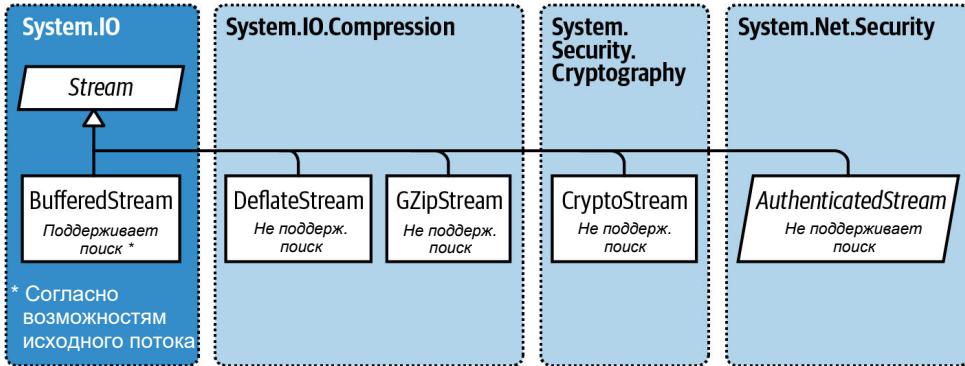
Рис. 15.4. Потоки с декораторами
