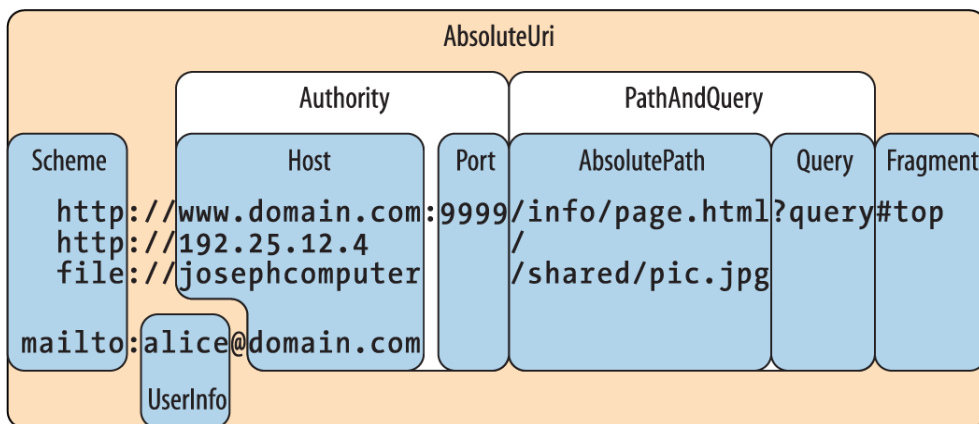
Рис. 16.2. Свойства класса Uri
