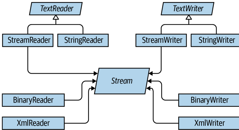
Рис. 15.5. Средства чтения и записи
