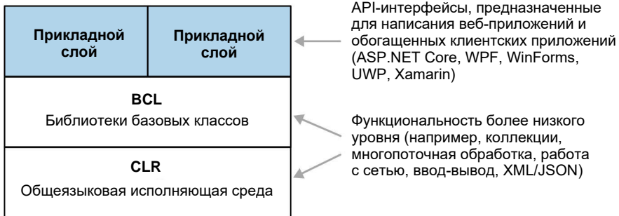
Рис. 1.1. Архитектура исполняющей среды
