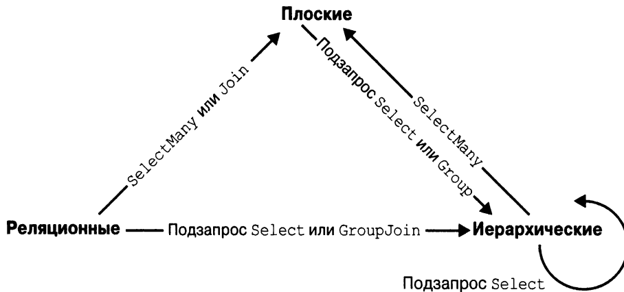
Рис. 9.1. Операции, изменяющие форму последовательностей
