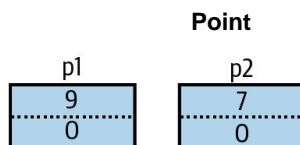
Рис. 2.2. Присваивание копирует экземпляр типа значения
