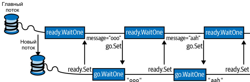
Рис. 21.2. Двухнаправленное сигналирование
