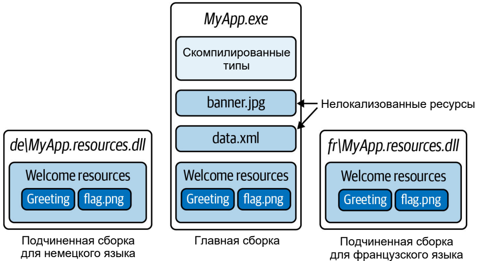
Рис. 17.2. Ресурсы
