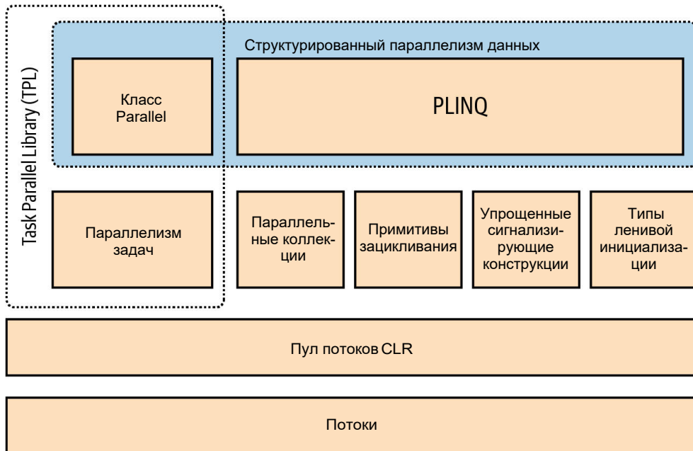
Рис. 22.1. Компоненты PFX
