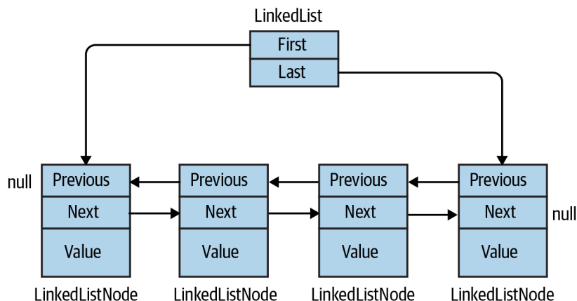
Рис. 7.4. Класс LinkedList<T>
