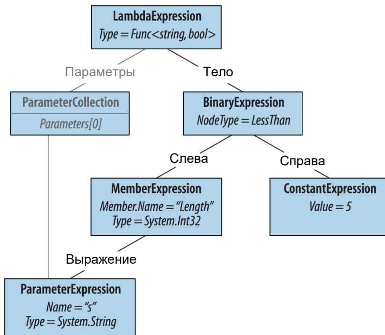
Рис. 8.11. Дерево выражения
