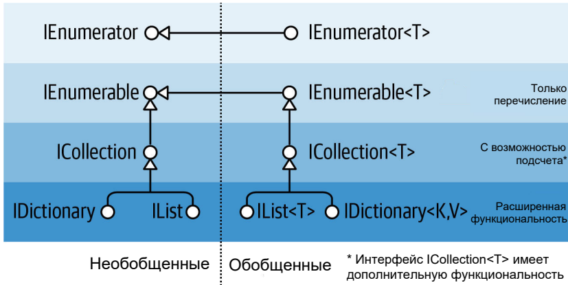
Рис. 7.1. Интерфейсы коллекций
