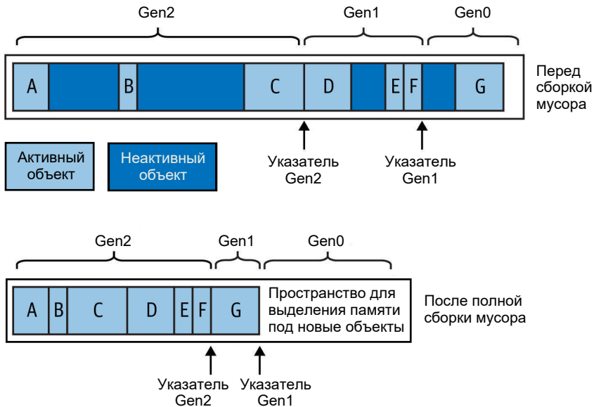
Рис. 12.2. Поколения кучи
