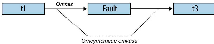
Рис. 22.6. Условные продолжения
