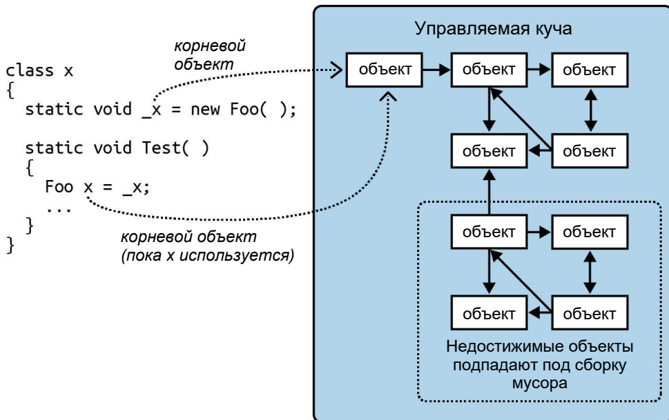
Рис. 12.1. Пример корневых объектов
