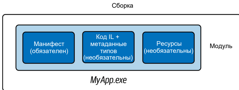
Рис. 17.1. Однофайловая сборка
