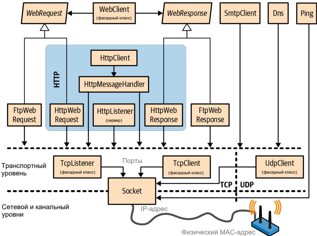
Рис. 16.1. Сетевая архитектура
