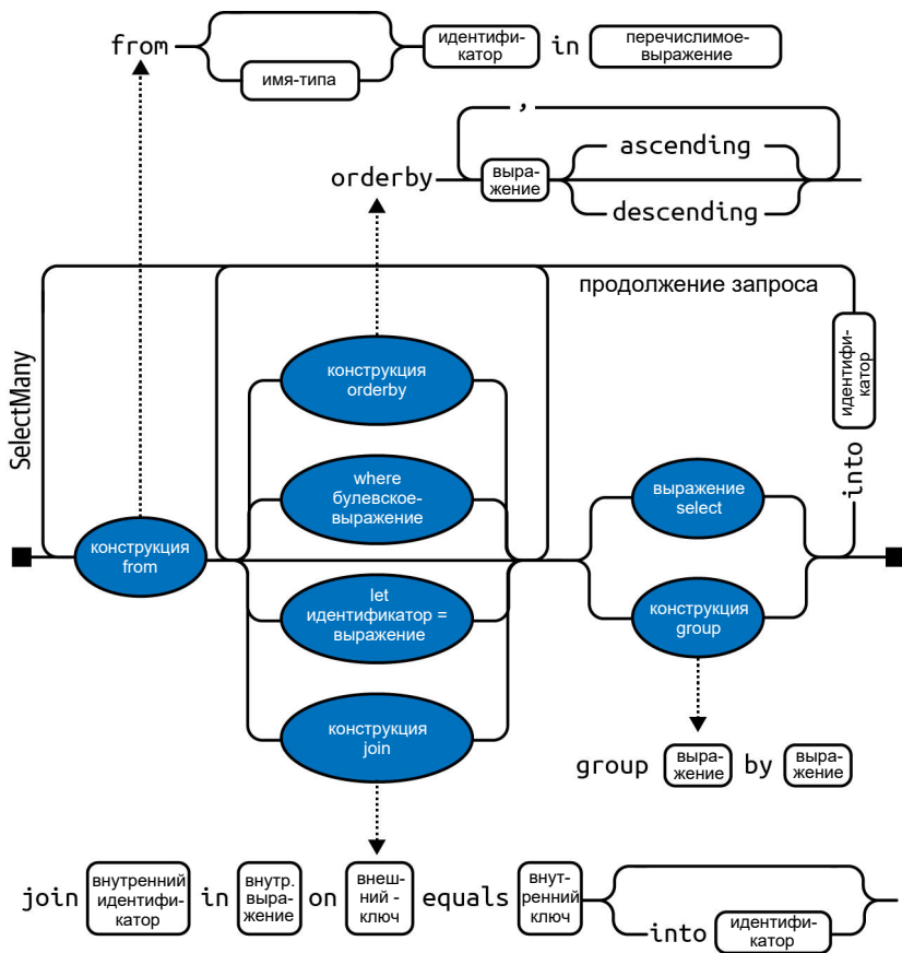
Рис. 8.2. Синтаксис запросов
