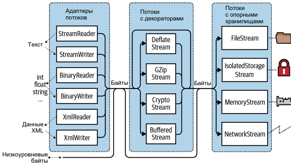
Рис. 15.1. Поточковая архитектура
