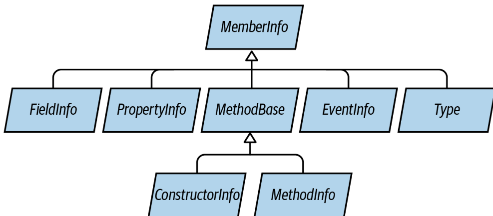
Рис. 18.1. Типы членов
