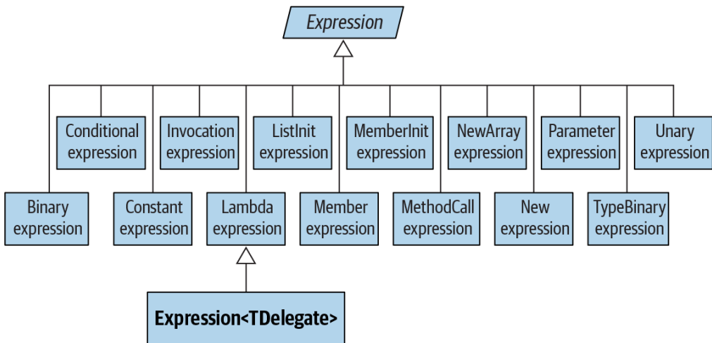
Рис. 8.10. Типы выражений
