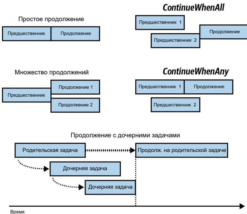
Рис. 22.5. Продолжения
