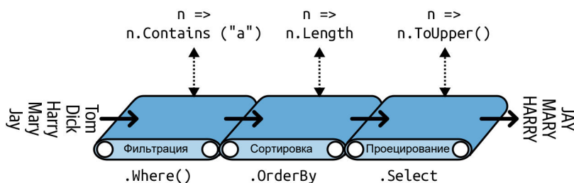
Рис. 8.1. Цепочка операций запросов
