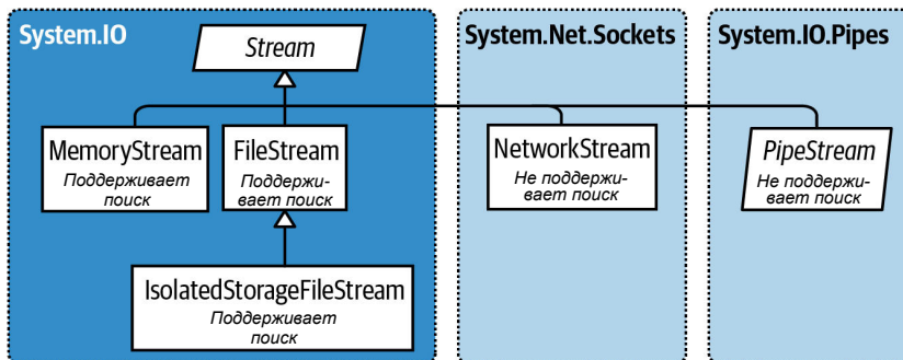
Рис. 15.2. Основные потоки с опорными хранилищами
