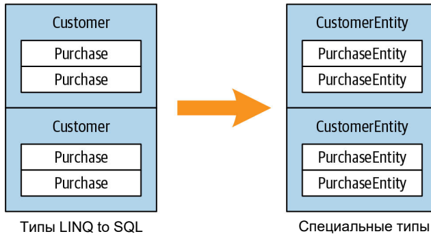
Рис. 9.2. Проецирование иерархии объектов
