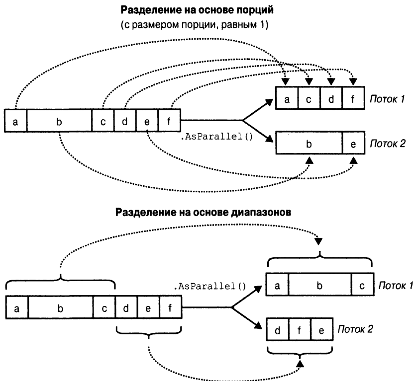
Рис. 22.4. Сравнение разбиения на основе порций и разбиения на основе диапазонов
