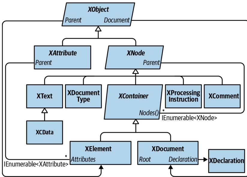
Рис. 10.1. Основные типы X-DOM
