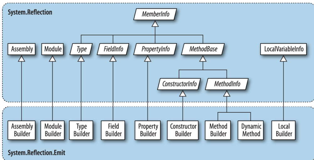
Рис. 18.2. Пространство имен System.Reflection.Emit
