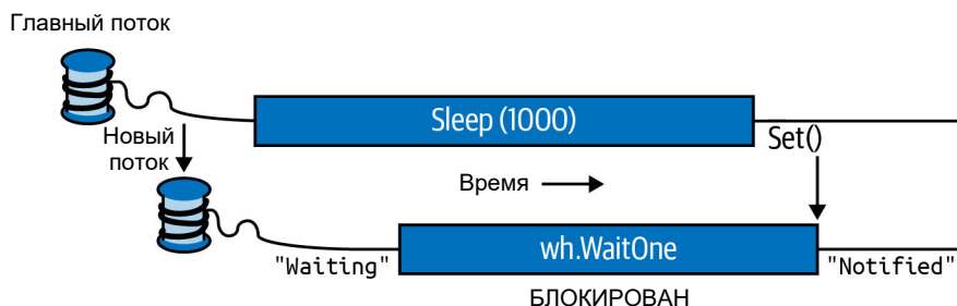
Рис. 21.1. Сигнализирование с помощью EventWaitHandle
