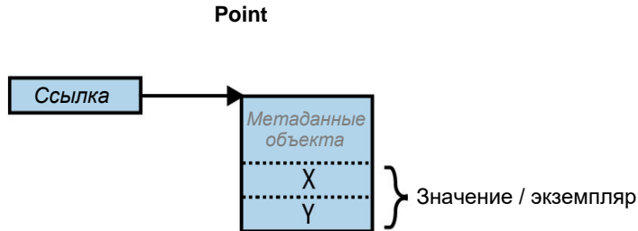
Рис. 2.3. Экземпляр ссылочного типа в памяти
