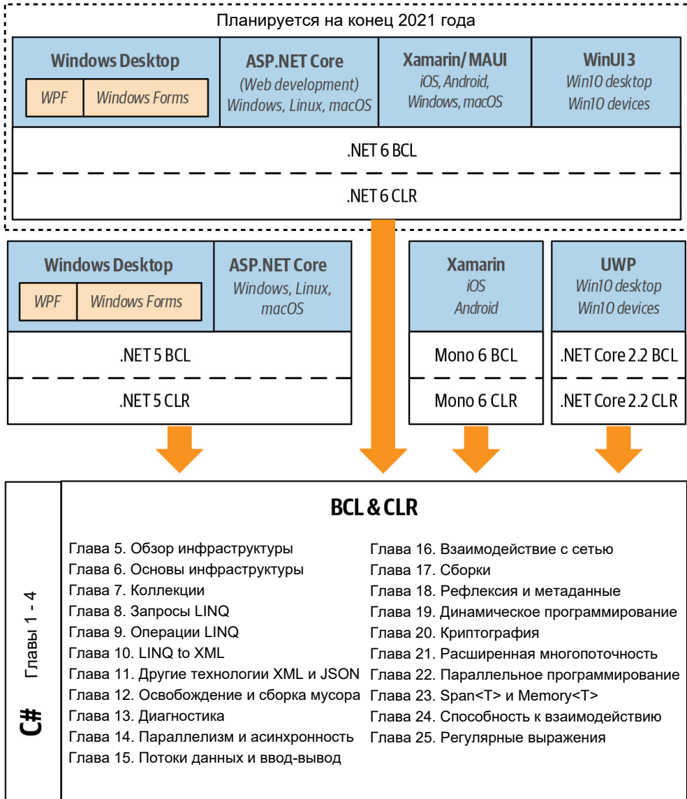
Рис. 1.2. Исполняющие среды для C#
