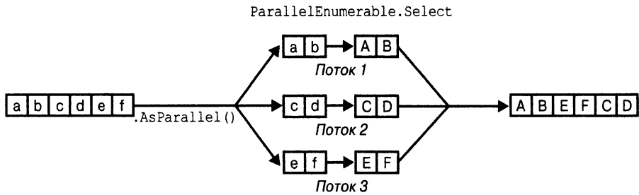
Рис. 22.2. Модель выполнения PLINQ
