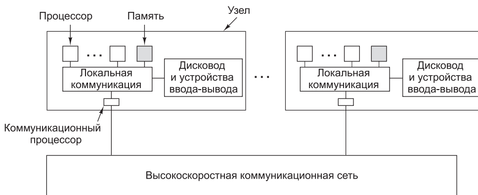
Рис. 8.32. Схема мультимьюльтикомпьютера
