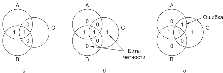
Рис. 2.11. Кодирование числа 1100 (а); добавляются биты четности (б); ошибка в секторе AC (в)
