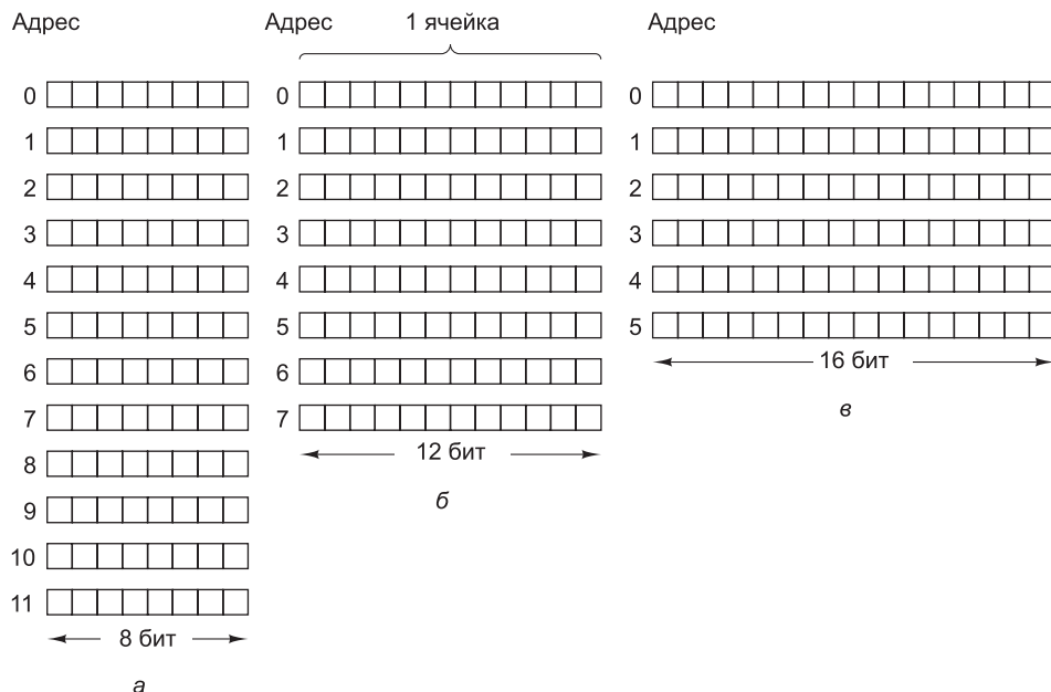
Рис. 2.8. Три варианта организации 96-разрядной памяти
