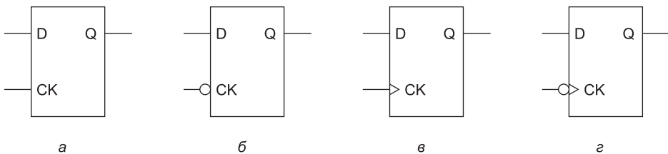
Рис. 3.25. D-защелки и D-триггеры
