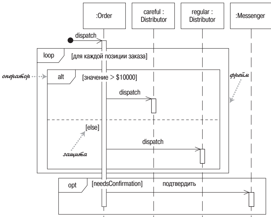
Рис. 4.4. Фреймы взаимодействия
