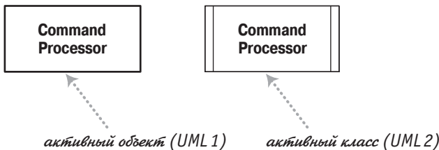
Рис. 5.21. Активный класс
