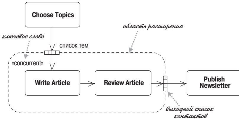
Рис. 11.9. Область расширения
