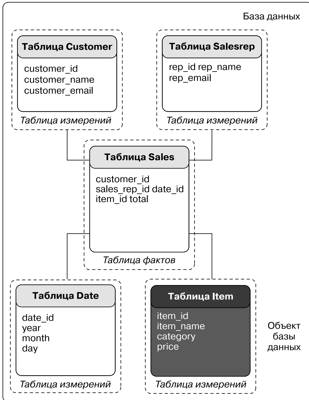
Рис. 5.1. База данных, содержащая схему «Звезда»
