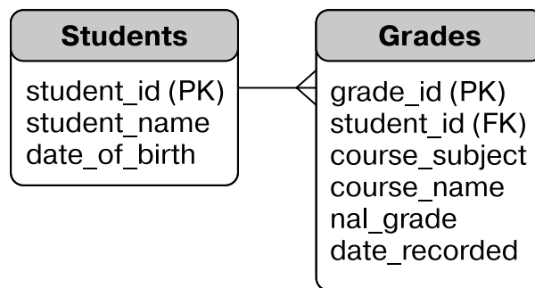
Рис. 1.3. Модель данных об оценках учащихся
