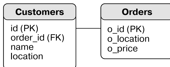
Рис. 5.2. Две таблицы с первичными ключами и внешним ключом
