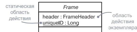
Рис. 9.4. Область действия
