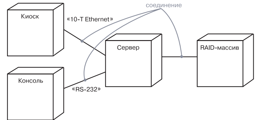
Рис. 27.4. Соединения
