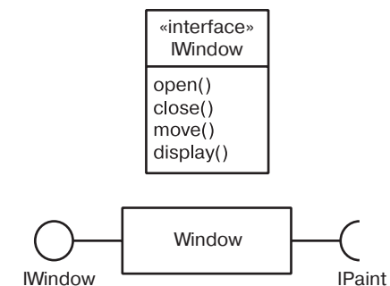
Рис. 2.2. Интерфейсы
