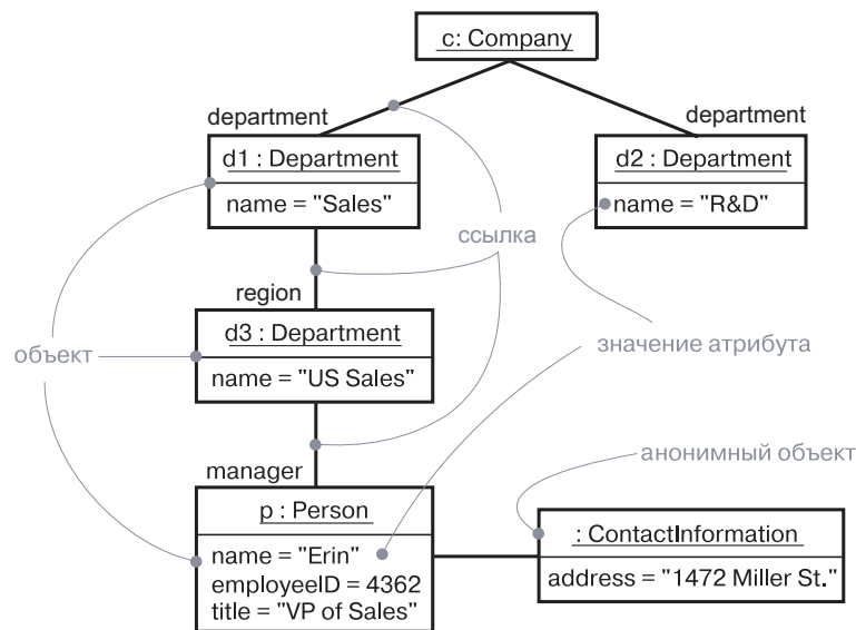
Рис. 14.1. Диаграмма объектов
