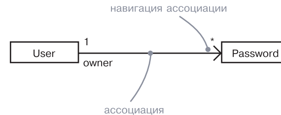
Рис. 10.3. Навигация
