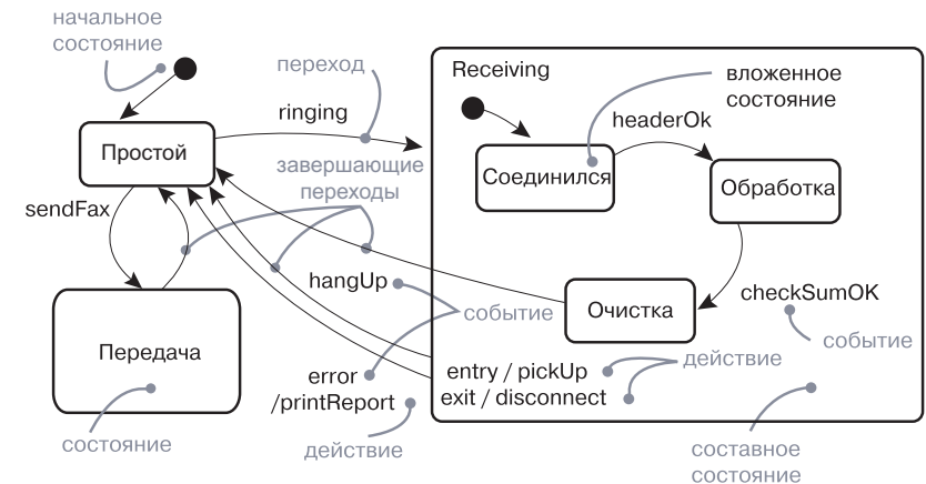
Рис. 25.1. Диаграмма состояний
