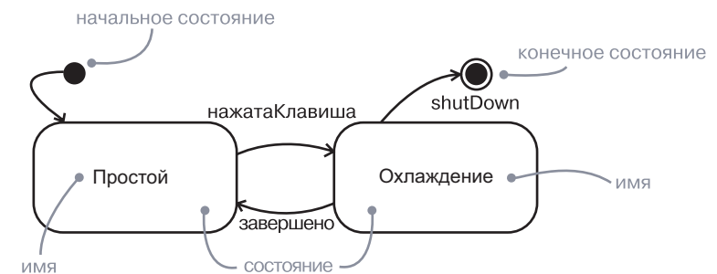
Рис. 22.2. Состояния
