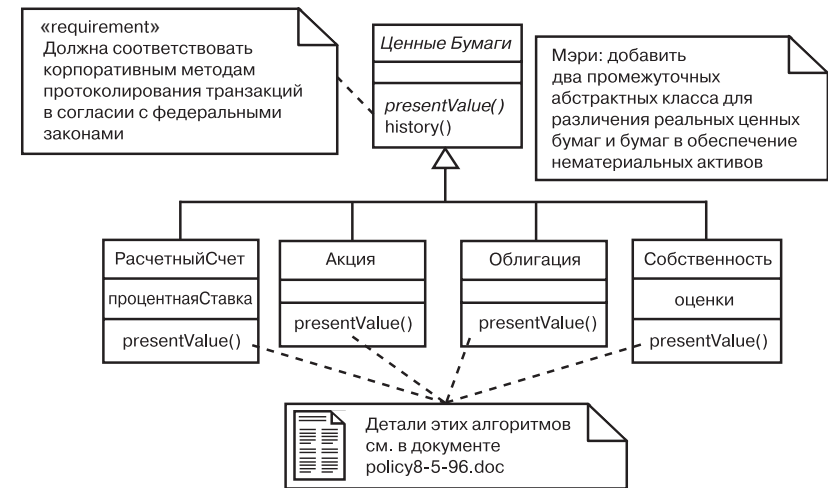
Рис. 6.9. Моделирование комментариев
