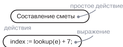
Рис. 20.2. Действия
