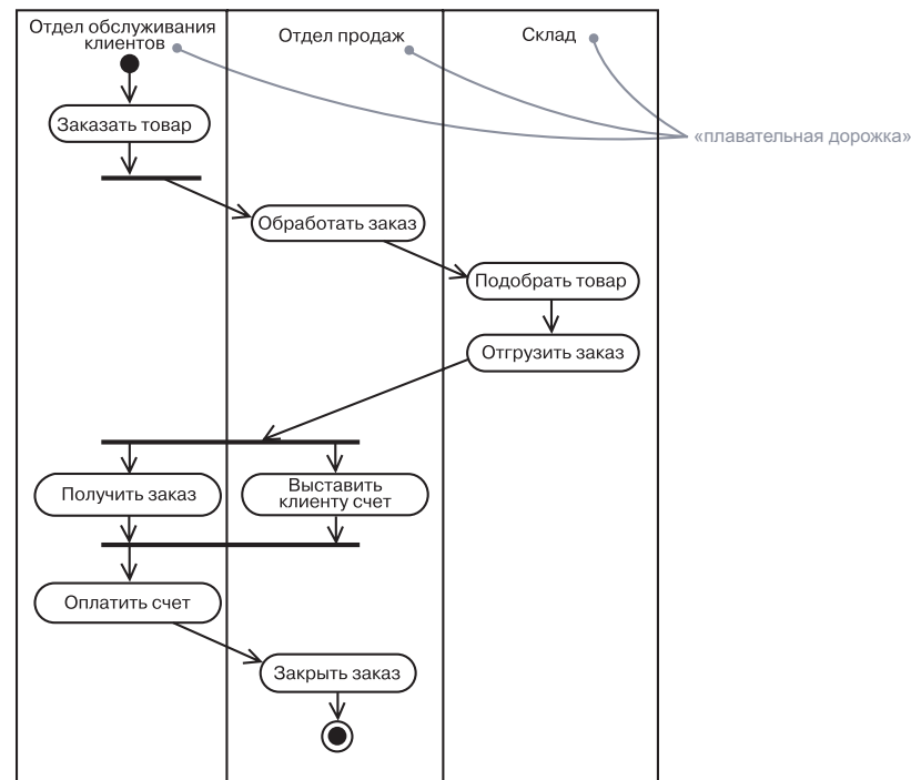
Рис. 20.7. «Плавательные дорожки»
