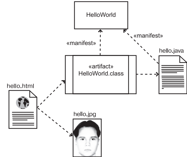
Рис. 3.6. Артефакты HelloWorld
