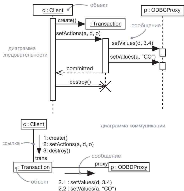
Рис. 19.1. Диаграммы взаимодействия
