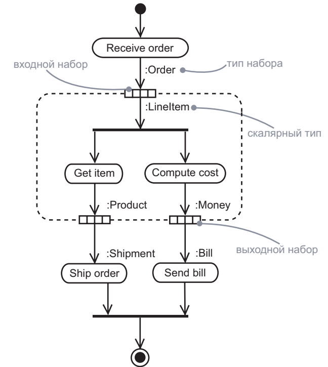
Рис. 20.9. Область расширения
