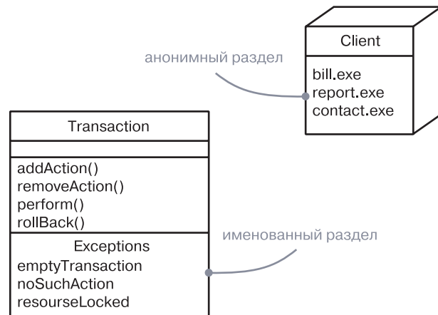
Рис. 6.4. Дополнительные разделы
