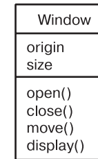
Рис. 2.1. Классы
