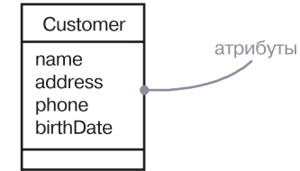
Рис. 4.3. Атрибуты
