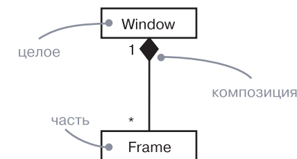
Рис. 10.6. Композиция
