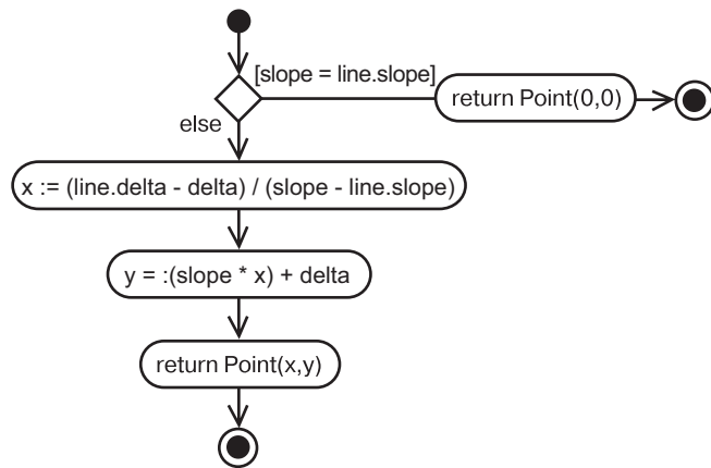
Рис. 20.11. Моделирование операции
