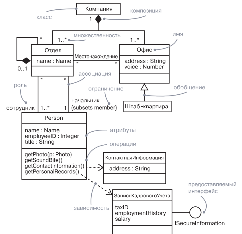
Рис. 8.1. Диаграмма классов
