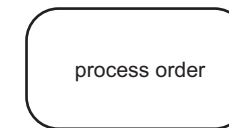
Рис. 2.11. Действия
