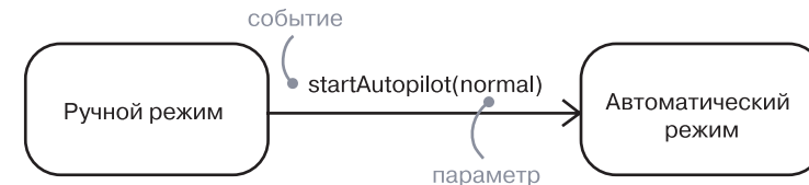
Рис. 21.3. События вызова
