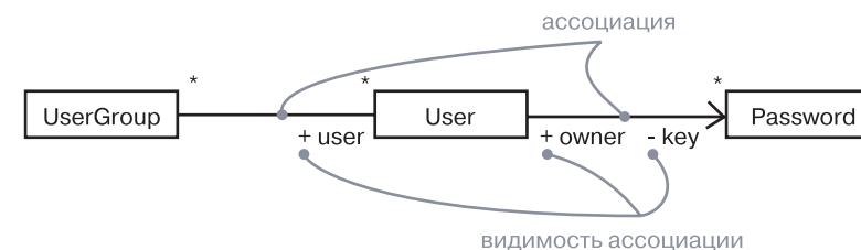
Рис. 10.4. Видимость
