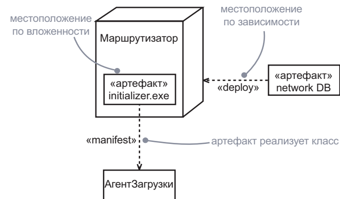
Рис. 24.3. Местоположение
