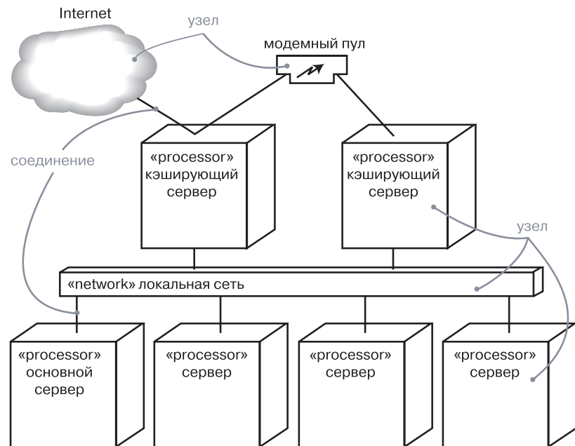
Рис. 31.1. Диаграмма размещения
