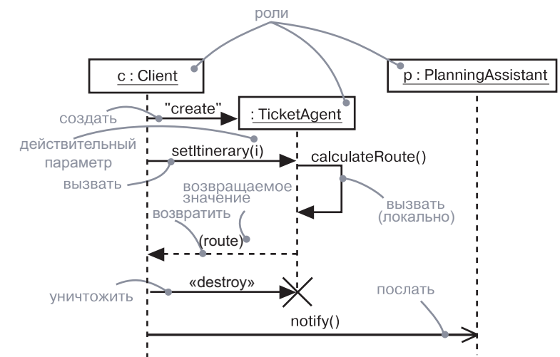
Рис. 16.3. Сообщения
