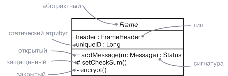
Рис. 9.1. Расширенные классы
