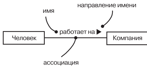
Рис. 5.4. Имена ассоциации
