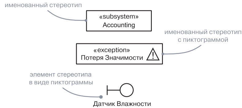
Рис. 6.5. Стереотипы
