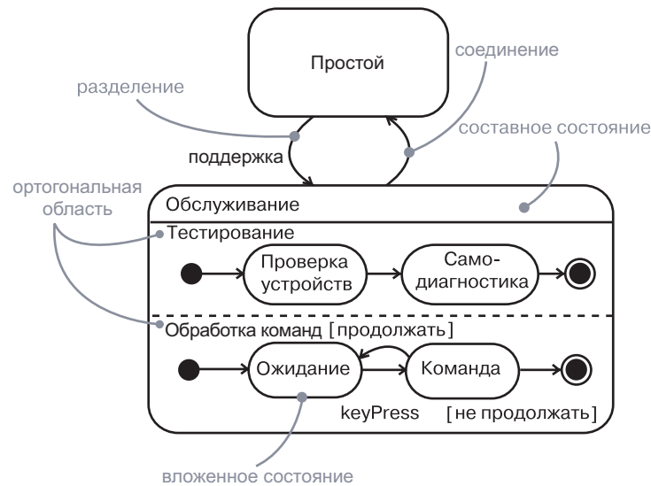
Рис. 22.7. Параллельные подсостояния
