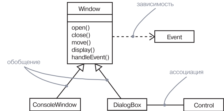
Рис. 5.1. Связи
