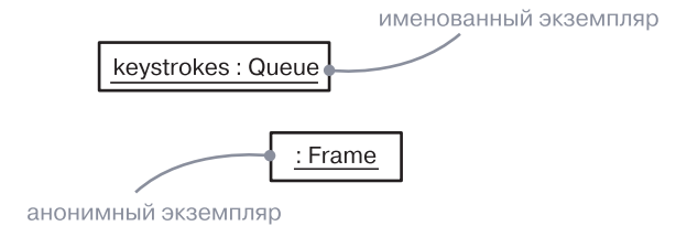
Рис. 13.1. Экземпляры
