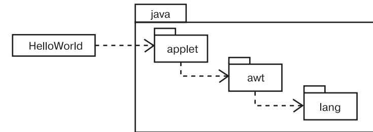
Рис. 3.4. Пакетирование HelloWorld
