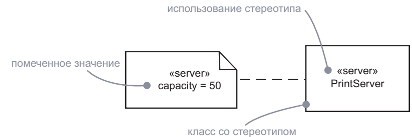
Рис. 6.7. Помеченные значения
