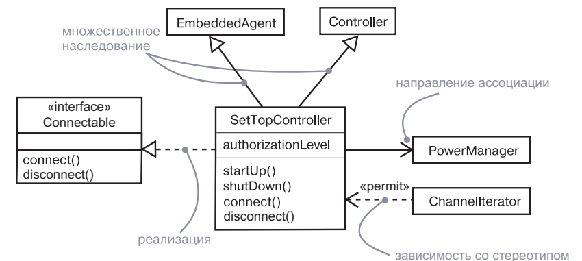
Рис. 10.1. Расширенные связи
