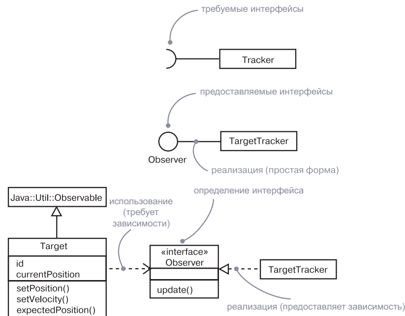
Рис. 11.4. Реализация
